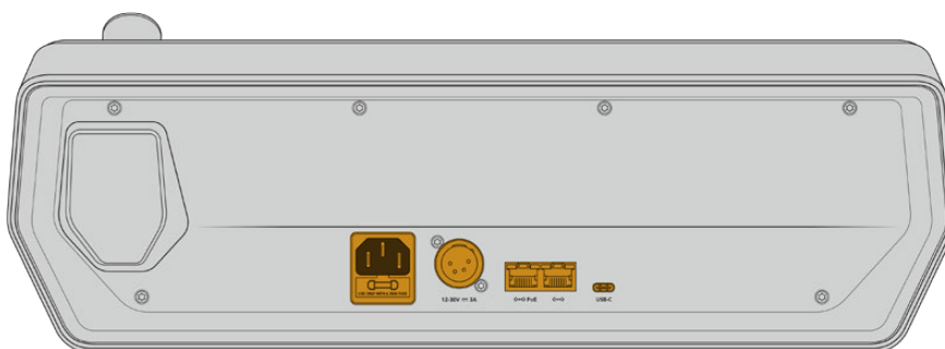
Разъемы на задней панели ATEM 1 M/E Advanced Panel
