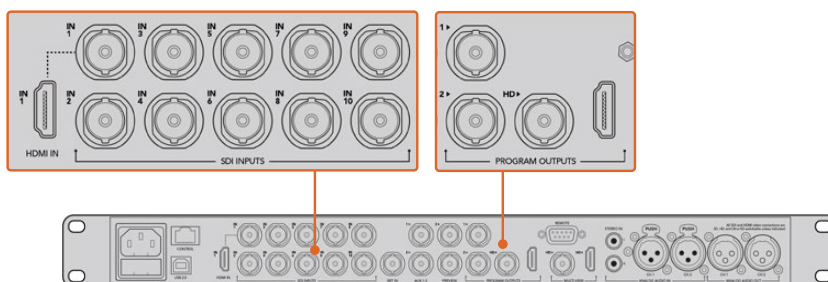
Conecte uma Blackmagic Studio Camera a qualquer uma das entradas SDI do switcher ATEM.
