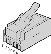
ATEM Constellation 8KのPTZリモート用RJ12ピン配列
