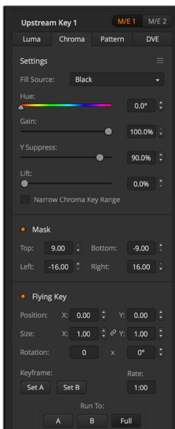
色键设置
