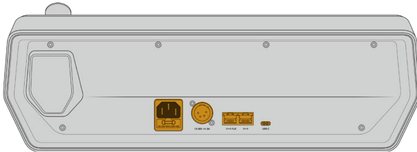
ATEM 1 M/E Advanced Panel 후면 연결
