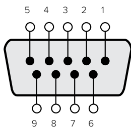
RS-422 PTZピン接続
