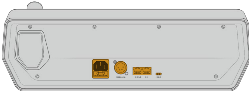
Conectores traseiros do ATEM 1 M/E Advanced Panel.
