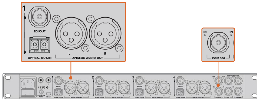
使用ATEM Studio Converter并通过光纤连接多台Blackmagic Studio Camera。 您需要为Studio Camera选购并安装SFP模块方可通过光纤接口连接。
